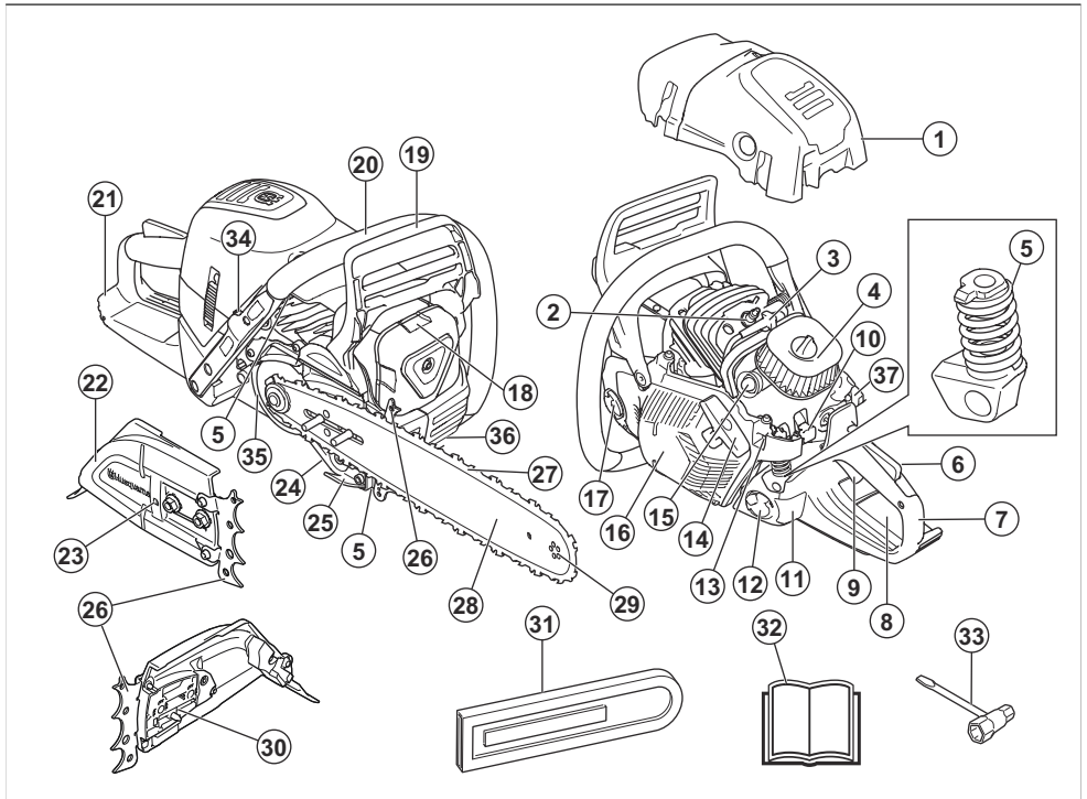
1. Sylinterikotelo
